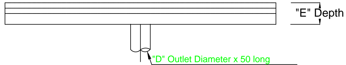
SECTION A-A HEELGUARD GRATE
