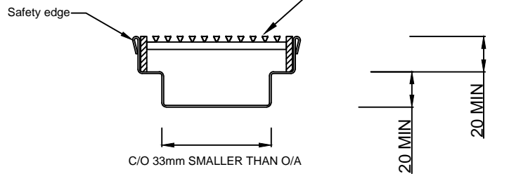
SECTION A-A HEELGUARD GRATE
